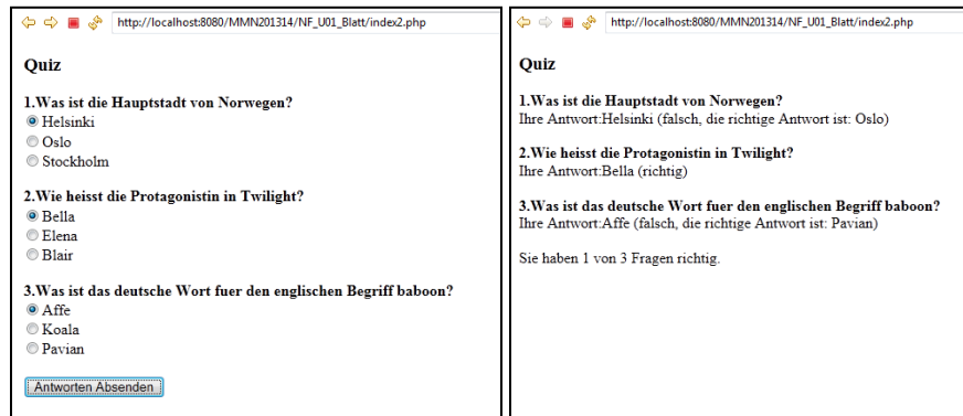
Abbildung 1: Screenshot einer möglichen Quiz-Anwendung. Der linke Screenshot zeigt die Fragen mit den Antwortmöglichkeiten. Der rechte Screenshot zeigt die Auswertung der eingereichten Lösungen.
