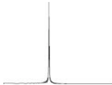
Sinus 110 Hz
