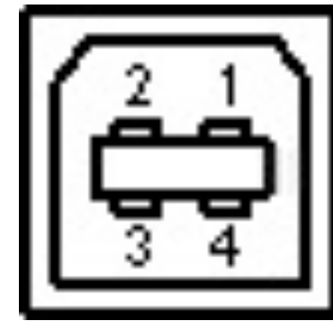
Type B USB connector Downstream (Gerät)
