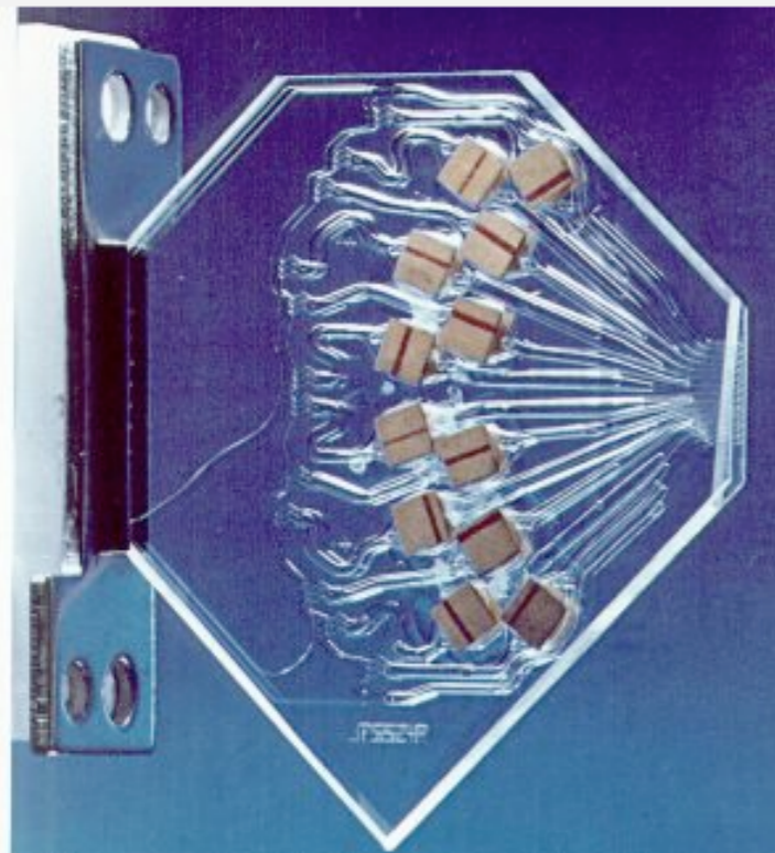
Glasgeätzter Piezo-Druckkopf (Epson 1985)
