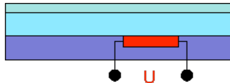
BubbleJet-Zelle als integrierte Schaltung (Canon, Xerox)
